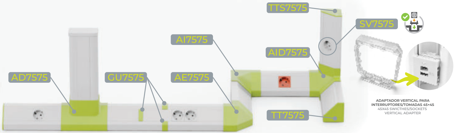
DERIVAÇÃO EM T (Ângulo Interior 90°) TEE ( Internal 90° Bend)
